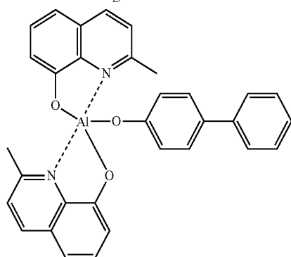
BAlq
