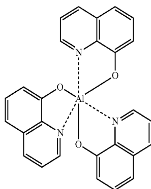
Alq 3
